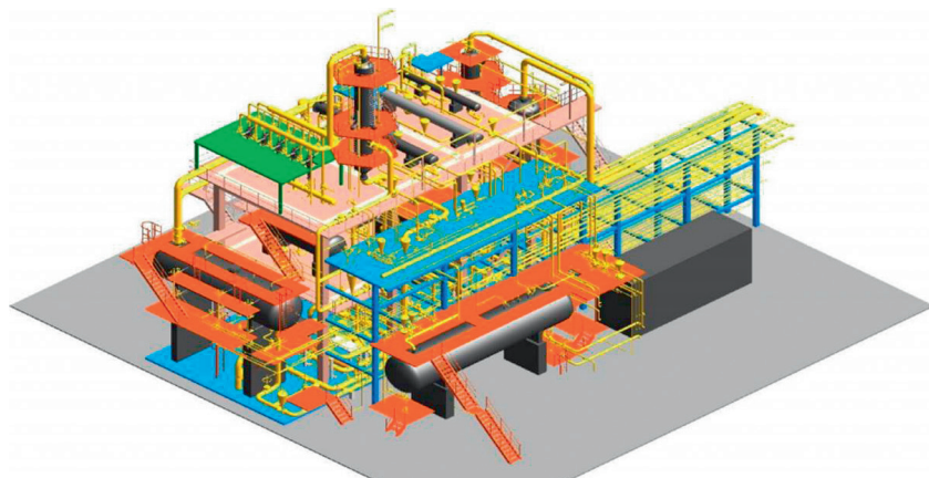
Установка 25/7 ОАО «Славнефть-Янос». Новый реакторный блок. 3D модель из программы AVEVA PDMS
